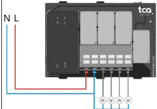
Figure 9: Schéma de câblage des bornes pour le mode volet roulant
