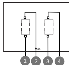
Figure 6: Configuration des sorties en mode éclairage avec volet roulant
