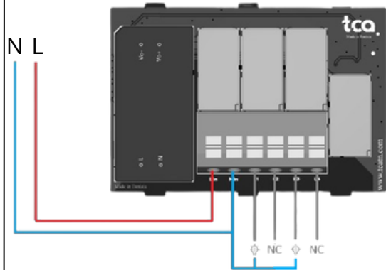
Figure 8: Schéma de câblage des bornes pour le mode éclairage
