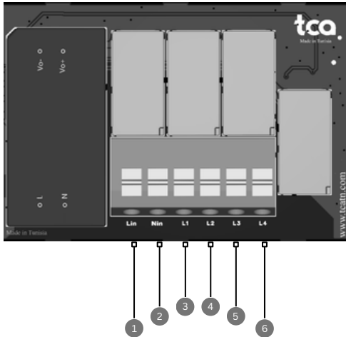
Figure 7: Schéma de câblage des bornes
